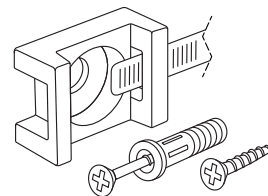
Платформа крепления, 2х Дюбель-гвоздь 6х40, 1х Саморез 4х30, 1х Хомут, 1х
